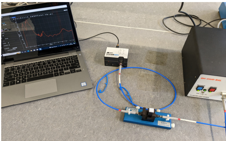
Abbildung 3: Das Spektrometer-Setup, welches durch die UniBern Forschungsstiftung finanziert wurde. Es zeichnet sich dadurch aus, dass es in rascher Reihenfolge (~150 Mal pro Sekunde) ein komplettes UV/VIS Spektrum aufnehmen kann. Die einzelnen Module (Lampe, Küvette, Detektor) sind mittels Glasfaserleitungen miteinander verbunden. Im installierten System befindet sich nur der Küvettenhalter in der Glove-Box.
